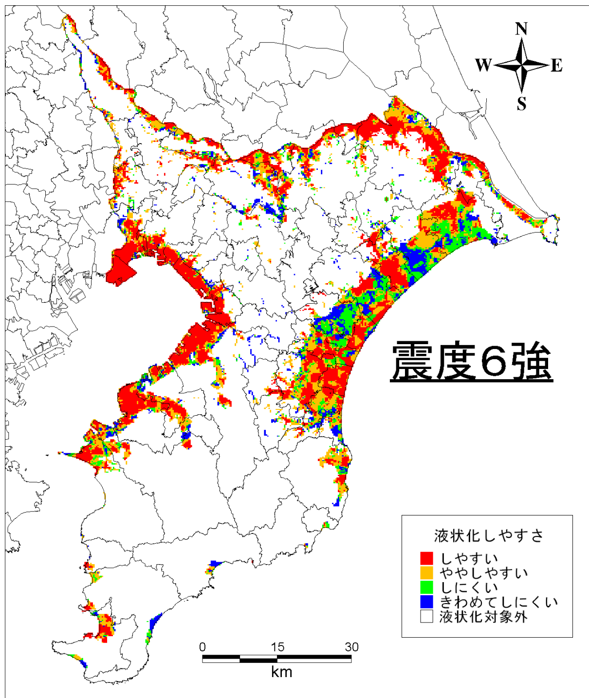
図 液状化しやすさマップ (直下地震・震度6強・地表加速度960gal)
